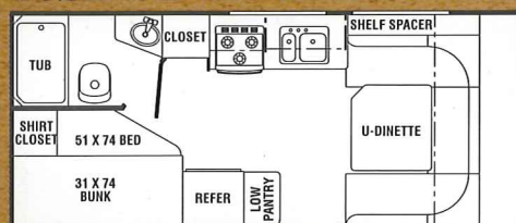
TC21RBH
