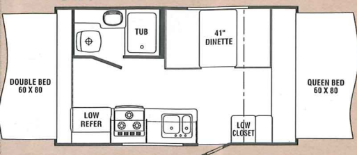
C17
