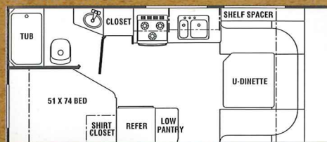
TC21DBL
